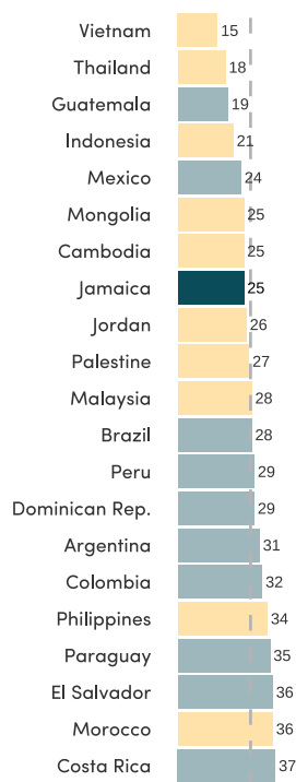
PISA 2022
