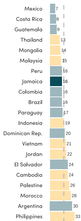
PISA 2022
